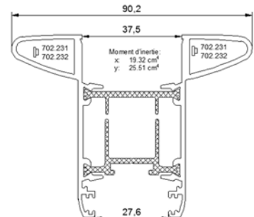
712.237 Montant ouvrant renforcé double petite tubulure galbée
