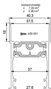
712.110 Traverse ouvrant
