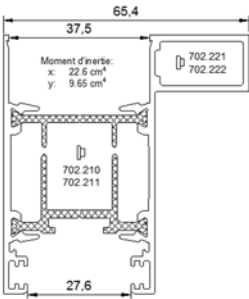
712.252 Montant ouvrant renforcé "sécuritaire"
