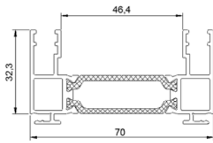
712-710 Dormant Montant c90 NT
