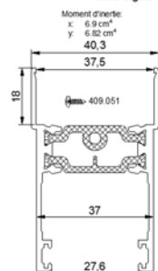
712.118 Traverse ouvrant sans ergots
