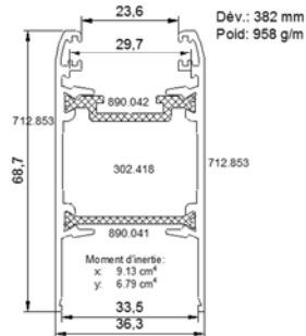
712-790 Montant simple
