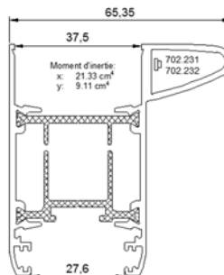
712.231 Montant ouvrant renforcé petite tubulure galbée
