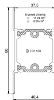
712.123 Traverse Intermediaire 80mm ouvrant 32mm
