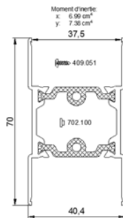
712.120 Traverse Intermediaire ouvrant
