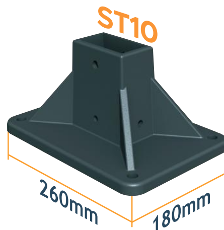
Encombre Platine de Fixation Platine standard
