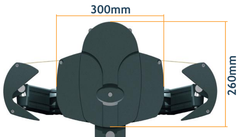
Encombre du Coffre Inclinaison 0° à 15°
