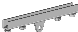
BSO4202 : Nb : 2 par travée Prémonté sur PBSO42 ( Pièce droite et gauche )
