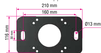
Support de fixation au sol ST45 Floor fixation support: ST45
