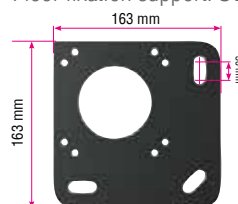
Support de fixation au sol : ST4502 Floor fixation support: ST4502
